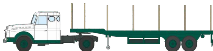
CB-191 - Camion WILLEME Tracteur couchette + Remorque à ridelles transport de bois
